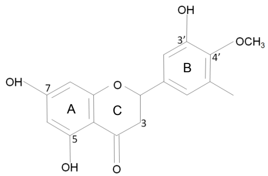
Hesperetin
