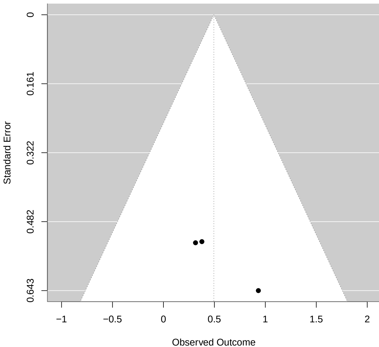
Funnel Plot: PANSS_Total_MA_FU
