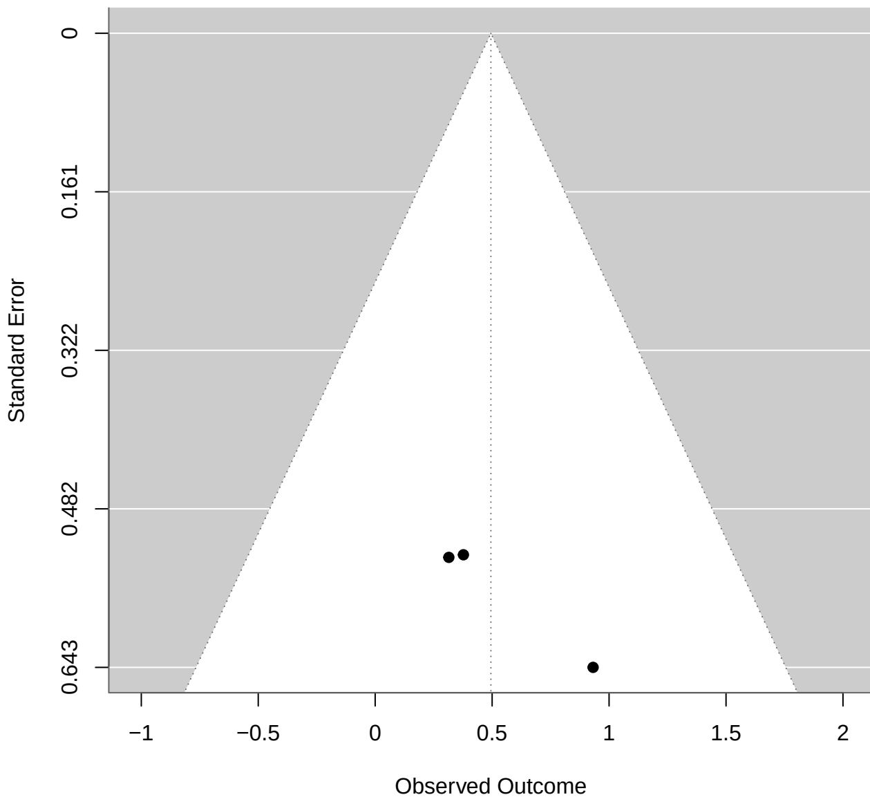
Funnel Plot: BDI_MA_FU
