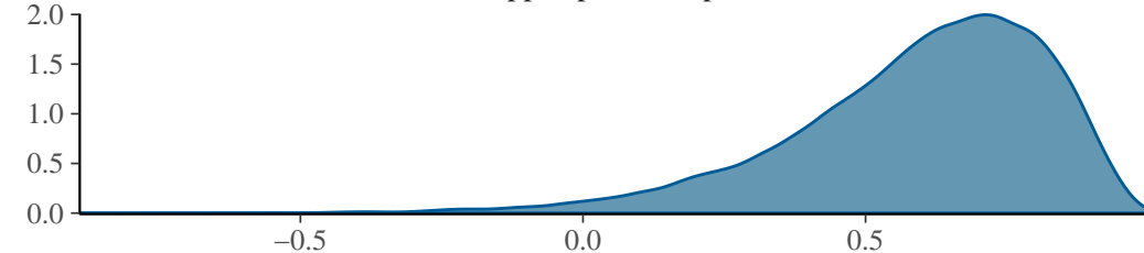
cor_id_ppts_pcseR_cpts_ccseR
