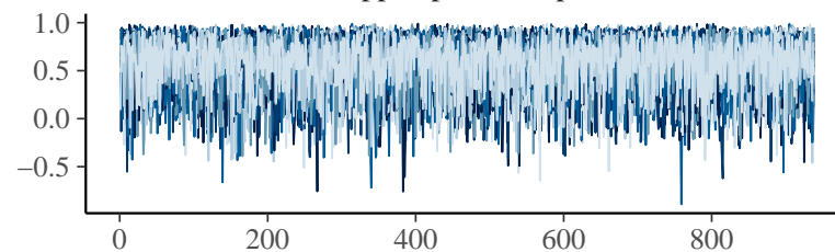
cor_id_ppts_pcseR_cpts_ccseR
